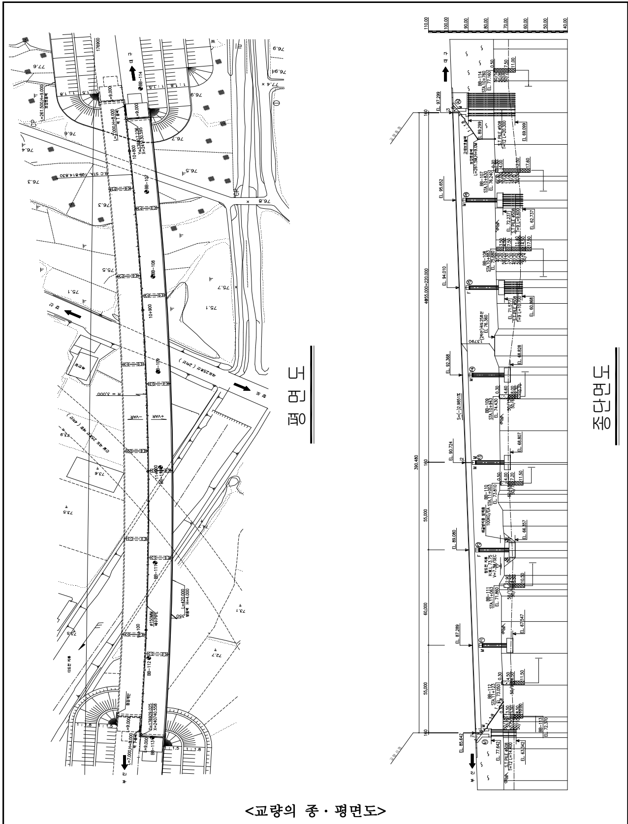
【그림 14.1】 송읍교 종·평면도
