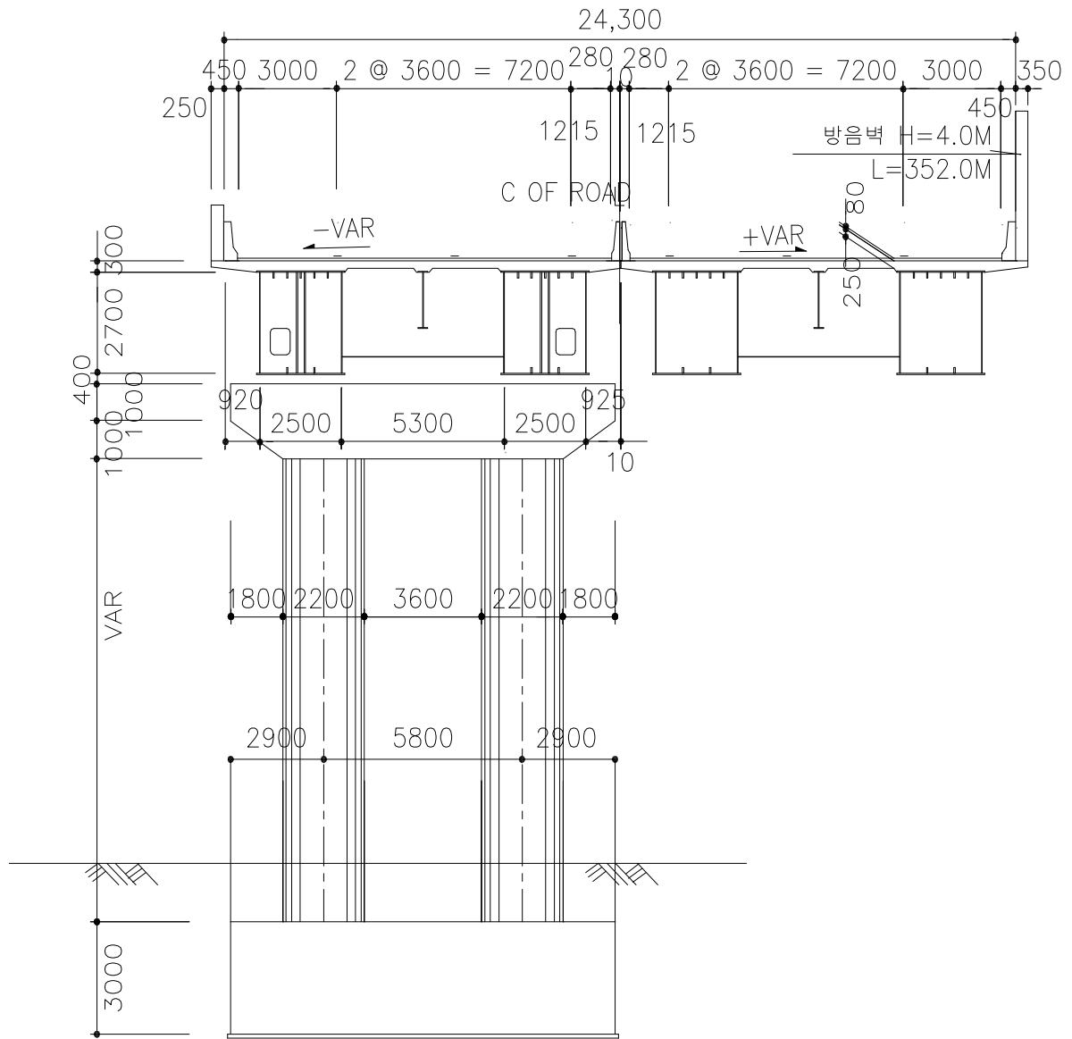
<횡단면도>
